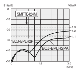
Return loss for BCJ-BPLH2P, BCJ-BPLH2PA
